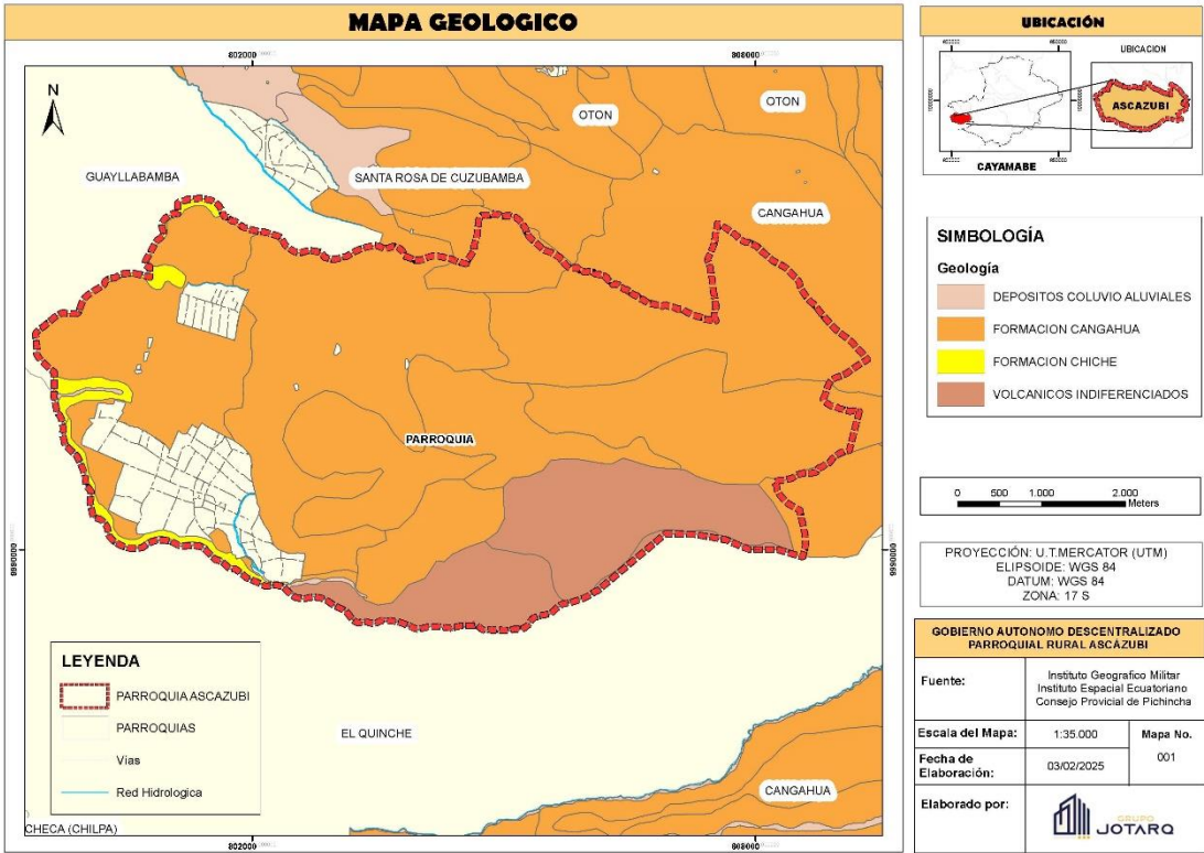
Ilustración 13 Mapa Geológico
